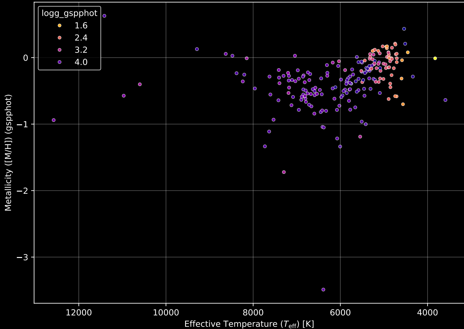
GALAH DR4 Field: [6783] Stellar Population Parameters (n= 201)
