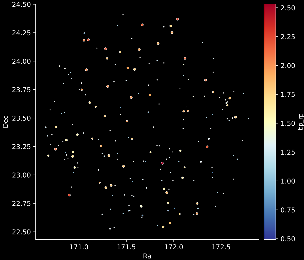
GALAH DR4 Field: [6783] Stars: 201
