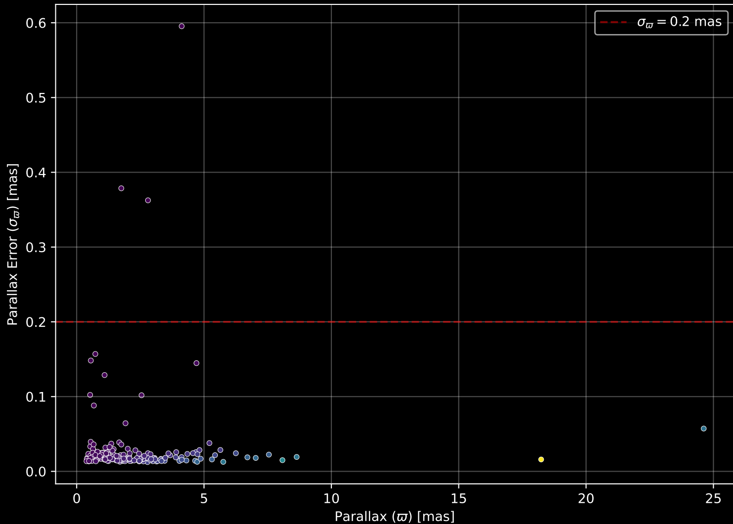
GALAH DR4 Field: [6783] Parallax Quality (n= 201)
