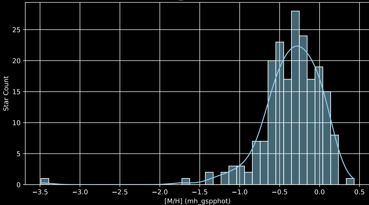
GALAH DR4 Field: [6783] [M/H] (mh_gspphot) (n= 200)
